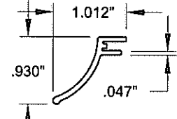
25 DRIP CAP #20021, 6063-T6
