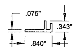
17 ADD-ON FIN/FLANGE #20008, Rigid PVC
