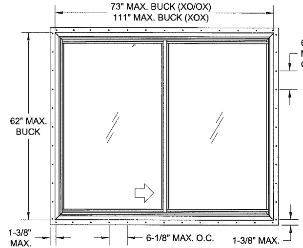
INTEGRAL FIN FRAME, XO
