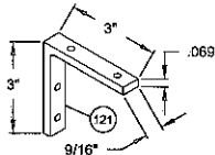
DETAIL 'L'
